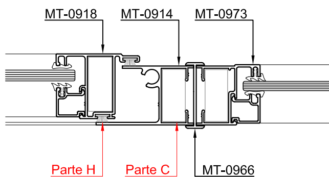
Corte 10-10
