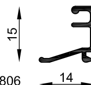
MT-0806 Contravidrio Peso estimado: 0.116 Kg/m Largo STD: 6030 mm
