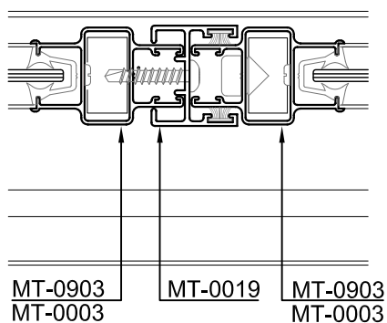
Encuentro 4 hojas
