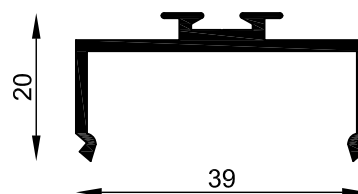
MT-0023 Tapa travesaño inferior Peso estimado: 0.362 Kg/m Largo STD: 6030 mm
