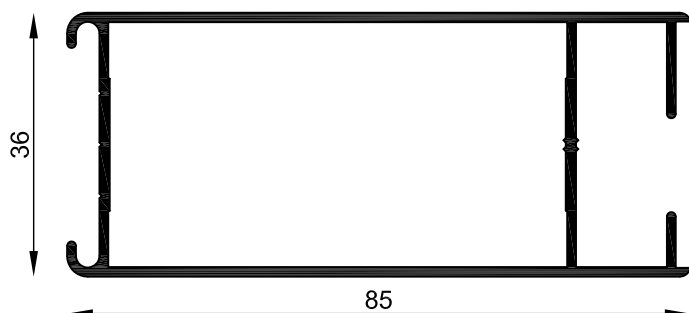
MT-0839 Parante puerta 36mm Peso estimado: 0.913 Kg/m Largo STD: 6150 mm
