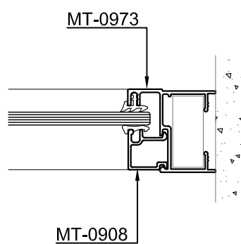
Corte 11-11
