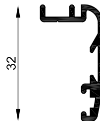
MT-2901 Contramarco Peso estimado: 0.259 Kg/m Largo STD: 6150 mm
