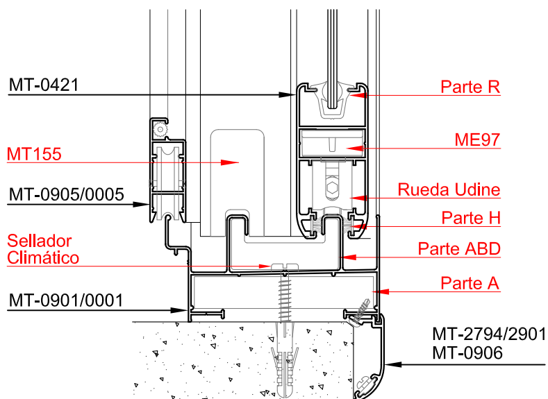
Corte 2-2
