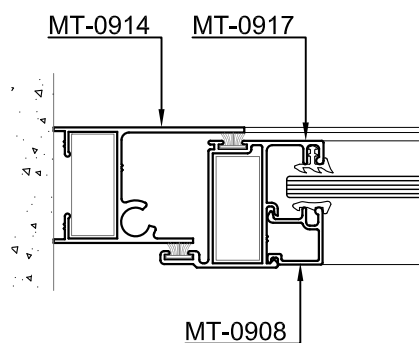
Corte 8-8
