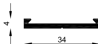
MT-2907 Tapajuntas puerta 44mm Peso estimado: 0.211 Kg/m Largo STD: 6150 mm
