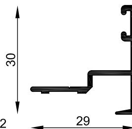
MT-2966 Marco de puerta 1,5" Peso estimado: 0.551 Kg/m Largo STD: 6150 mm
