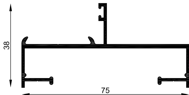
MT-0524 Marco puerta de rebatir bisagra encolizada Peso estimado: 0.672 Kg/m Largo STD: 6150 mm
