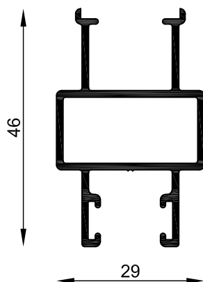
MT-0003 Parante lateral hoja corrediza Peso estimado: 0.564 Kg/m
