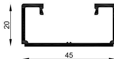
MT-2765 Adaptador celosía regulable Peso estimado: 0.435 Kg/m Largo STD: 6030 mm
