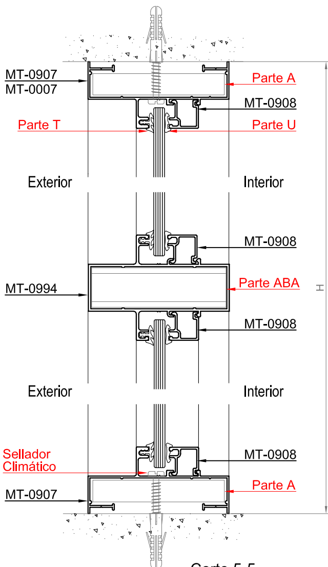
Corte 5-5
