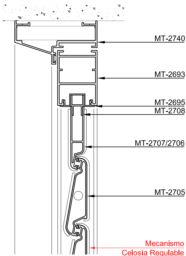
Corte 11-11
