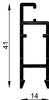
MT-0005 Marco mosquitero Peso estimado: 0.408 Kg/m Largo STD: 6030 mm
