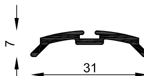
MT-0815 Tapacanto vaivén Peso estimado: 0.189 Kg/m Largo STD: 6030 mm
