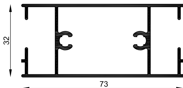
MT-0840 Travesaño puerta Peso estimado: 0.926 Kg/m Largo STD: 6030 mm
