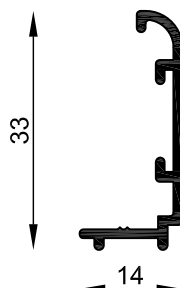
MT-0829 Contramarco Peso estimado: 0.197 Kg/m Largo STD: 6030 mm
