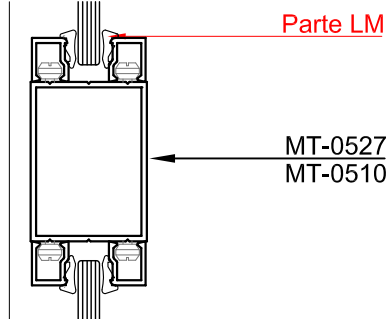
Corte 8"-8"
