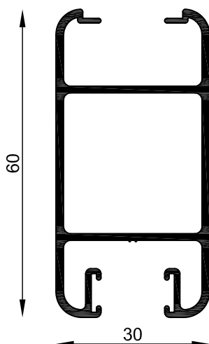
MT-0853 Parante lateral reforzado Peso estimado: 0.829 Kg/m Largo STD: 6150 mm
