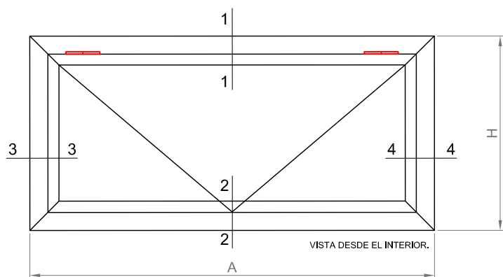
B- Ventiluz
