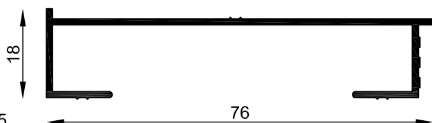
MT-0825 Premarco simple 75mm Peso estimado: 0.429 Kg/m Largo STD: 6150 mm
