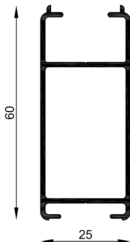
MT-0978 Batiente reforzado postigón Peso estimado: 0.583 Kg/m Largo STD: 6150 mm
