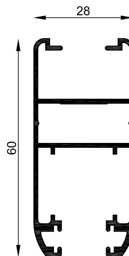
MT-0421 Umbral y dintel de Hoja Peso estimado: 0.729 Kg/m Largo STD: 6030 mm
