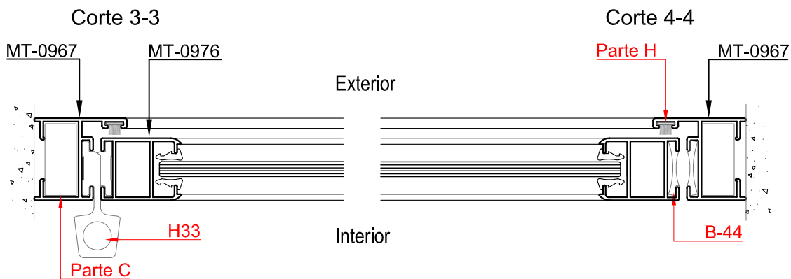
Corte 3-3
