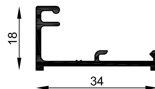
MT-0925 Porta contravidrio simple Peso estimado: 0.251 Kg/m Largo STD: 6030 mm
