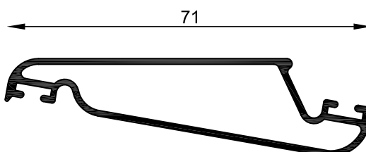
MT-2705 Tablilla celosía regulable Peso estimado: 0.529 Kg/m Largo STD: 6030 mm
