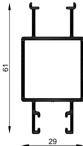
MT-0053 Parante lateral hoja corrediza Peso estimado: 0.694 Kg/m Largo STD: 6150 mm
