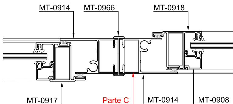
Corte 9-9
