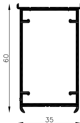
MT-0509 Hoja puerta de rebatir Peso estimado: 0.840 Kg/m Largo STD: 6030 mm
