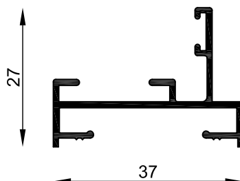
MT-0846 Marco de postigón para puerta Peso estimado: 0.335 Kg/m Largo STD: 6150 mm
