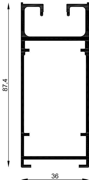
MT-2682 Batiente ancho puerta 36 mm Peso estimado: 1.207 Kg/m Largo STD: 6030 mm
