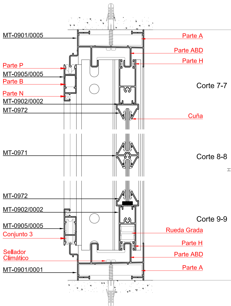
Encuentro 4 hojas
