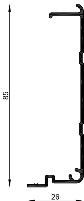
MT-0922 Soporte Tapa cinta Peso estimado: 0.478 Kg/m Largo STD: 6030 mm
