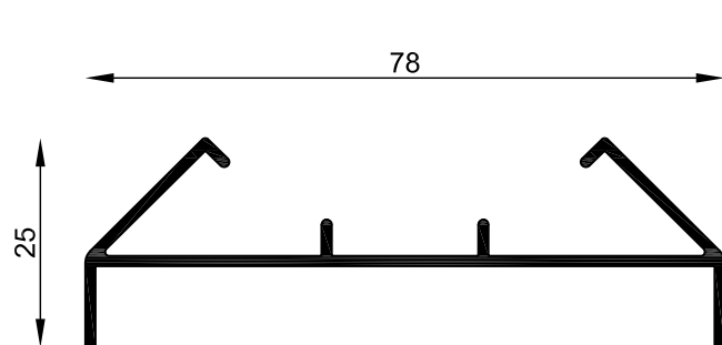
MT-0187 Apoyo rótula Peso estimado: 0.518 Kg/m Largo STD: 6030 mm
