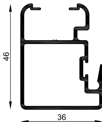
MT-0854 Parante central reforzado moderno Peso estimado: 0.726 Kg/m Largo STD: 6150 mm
