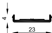
MT-2690 Base moldura puerta placa Peso estimado: 0.116 Kg/m Largo STD: 6030 mm
