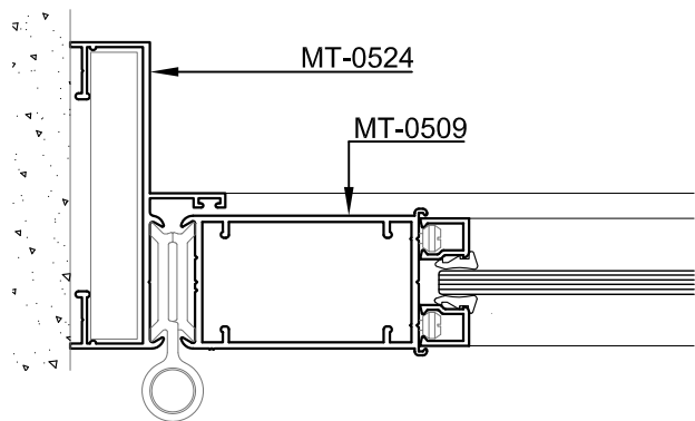
Corte 10"-10"
