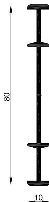
MT-0049 Acople tapajunta 75mm Peso estimado: 0.518 Kg/m Largo STD: 6030 mm
