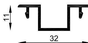
MT-2695 Adaptador terminal celosía regulable Peso estimado: 0.173 Kg/m Largo STD: 6030 mm
