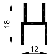
MT-2708 Calce tapaluz celosía regulable Peso estimado: 0.151 Kg/m Largo STD: 6030 mm
