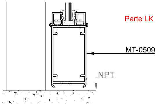
Corte 9"-9"
