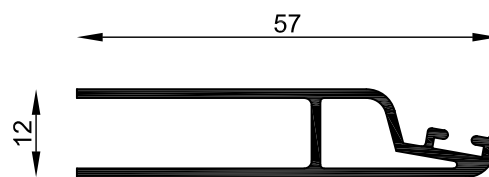
MT-2707 Terminal largo celosía regulable Peso estimado: 0.448 Kg/m Largo STD: 6030 mm
