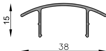
MT-0894 Tapa Peso estimado: 0.189 Kg/m Largo STD: 6030 mm
