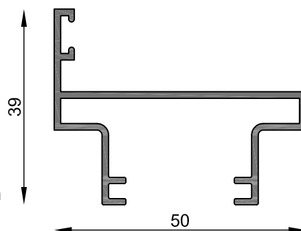
MT-0893 Marco puerta tabique Peso estimado: 0.513 Kg/m Largo STD: 6150 mm
