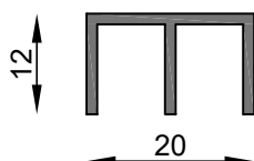
MT-1674 Dintel vitrina Peso estimado: 0.184 Kg/m Largo STD: 6030 mm
