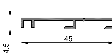
MT-1396 Tapa dintel tabique divisorio Peso estimado: 0.216 Kg/m Largo STD: 6030 mm
