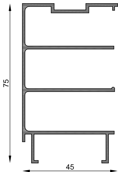
MT-0190 Zócalo tabiquería tubular Peso estimado: 0.996 Kg/m Largo STD: 6030 mm
