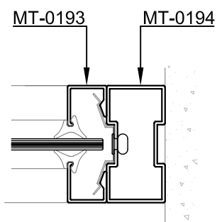
Corte 9-9
