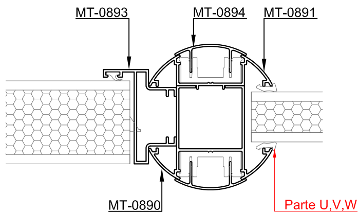
Corte 11-11
