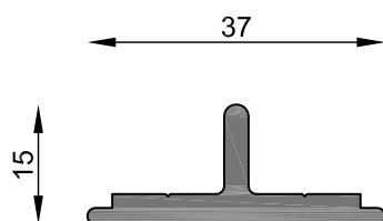
MI-0135 Presilla de hoja fija PRE-950 Peso estimado: 0.424 Kg/m Largo STD: 6030 mm
