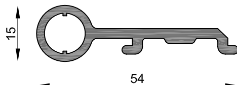
MT-1127 Bisagra Peso estimado: 0.605 Kg/m Largo STD: 6030 mm
