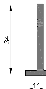
MT-1952 Porta rueda cubre bañera Peso estimado: 0.321 Kg/m Largo STD: 6030 mm
