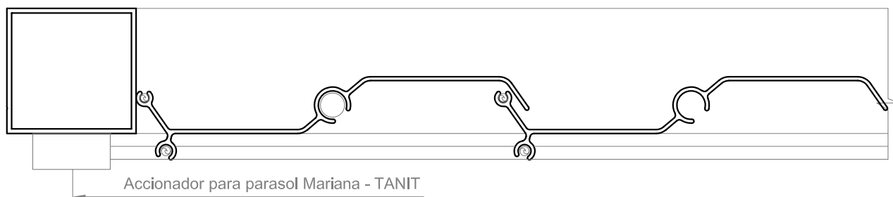
CORTE 1-1
