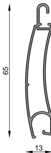
MT-0991 Tablilla de Cortina Peso estimado: 0.424 Kg/m Largo STD: 6030 mm
