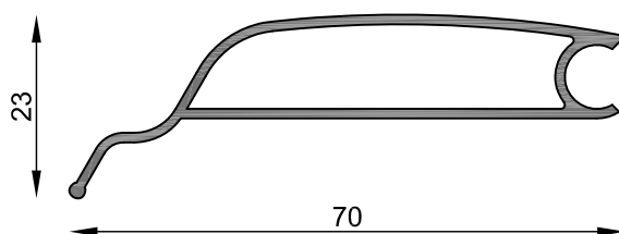
MT-2701 Primera tablilla cortina regulable Peso estimado: 0.475 Kg/m Largo STD: 6030 mm
