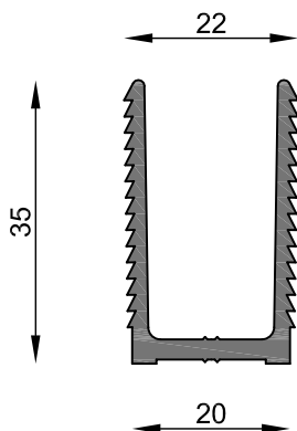
MT-0479 "U" de armado Peso estimado: 0.489 Kg/m Largo STD: 6030 mm
