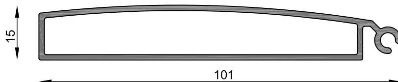
MT-2700 Zócalo cortina regulable Peso estimado: 0.894 Kg/m Largo STD: 6030 mm
