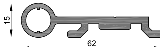
MT-0844 Bisagra Peso estimado: 0.818 Kg/m Largo STD: 6030 mm
