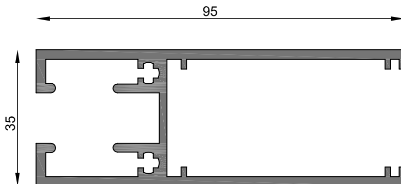
MT-0564 Umbral - vidrio temp. Peso estimado: 1.866 Kg/m Largo STD: 6030 mm
