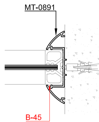
Corte 9-9
