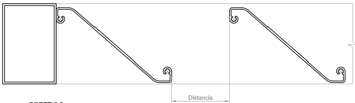
CORTE 2-2
