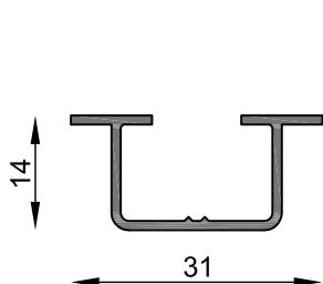
MT-0895 Porta vidrio Peso estimado: 0.197 Kg/m Largo STD: 6030 mm
