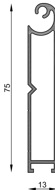
MT-2852 Zocalo cortina de enrollar Peso estimado: 0.643 Kg/m Largo STD: 6030 mm
