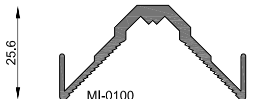
MI-0100 Escuadra para premarco Peso estimado: 0.543 Kg/m Largo STD: 6030 mm
