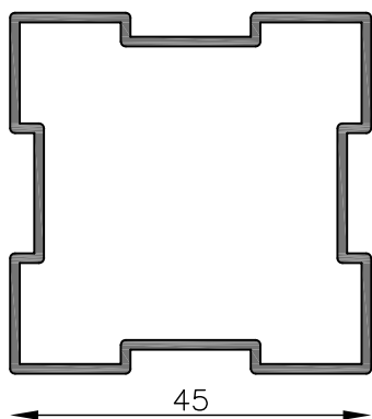
MT-0195 Columna tabiquería tubular Peso estimado: 0.640 Kg/m Largo STD: 6030 mm
