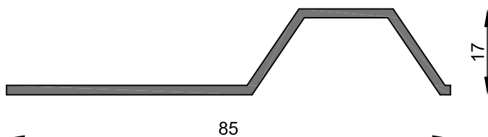
MI-0138 Soporte para MT127 Peso estimado: 0.486 Kg/m Largo STD: 6030 mm
