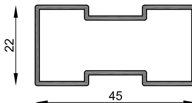
MT-0194 Travesaño tabiquería tubular Peso estimado: 0.459 Kg/m Largo STD: 6030 mm
