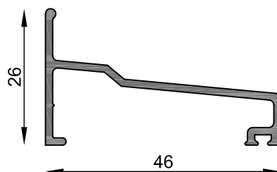
MT-1349 Umbral sanitario cubre bañera Peso estimado: 0.348 Kg/m Largo STD: 6030 mm
