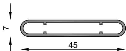
MT-0802 Tablilla celosia Peso estimado: 0.302 Kg/m Largo STD: 6030 mm
