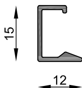
MT-0192 Contravidrio corto Peso estimado: 0.111 Kg/m Largo STD: 6030 mm
