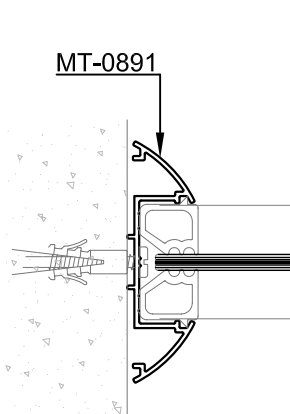
Corte 7-7
