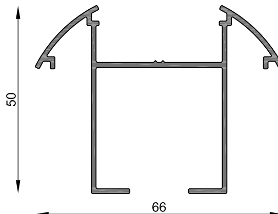
MT-0890 Columna Peso estimado: 0.680 Kg/m Largo STD: 6030 mm
