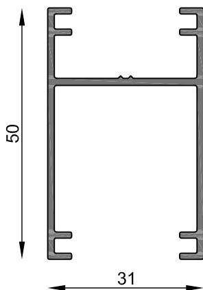
MT-0892 Travesaño Peso estimado: 0.548 Kg/m Largo STD: 6030 mm
