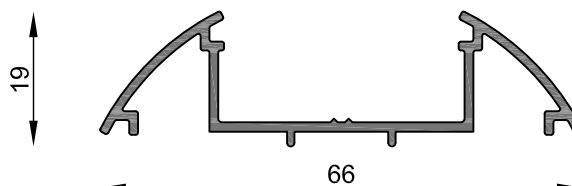
MT-0891 Tapa columna Peso estimado: 0.416 Kg/m Largo STD: 6030 mm
