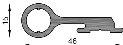
MT-0843 Bisagra Peso estimado: 0.610 Kg/m Largo STD: 6030 mm
