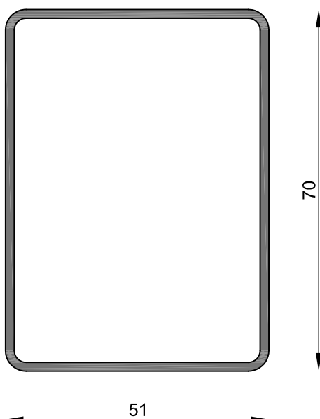
MT-5401 Empalme de columna LUV 974 Peso estimado: 1.061 Kg/m Largo STD: 6000 mm
