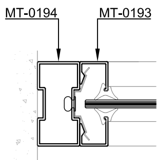
Corte 7-7
