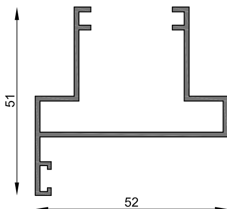
MT-1393 Parante 50 mm Peso estimado: 0.616 Kg/m Largo STD: 6150 mm
