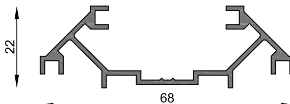
MT-1392 Tapa columna tabique divisorio Peso estimado: 0.537 Kg/m Largo STD: 6030 mm
