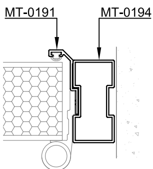
Corte 12-12
