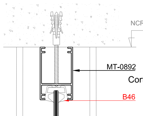
Corte 1-1
