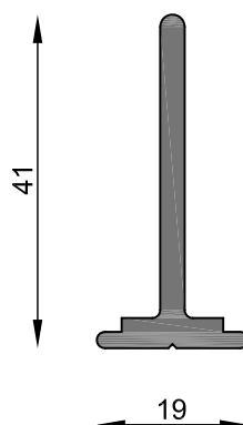
MI-0137 Presilla para hoja fija PRE-951 Peso estimado: 0.456 Kg/m Largo STD: 6030 mm
