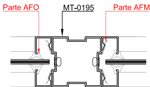
Corte 8-8
