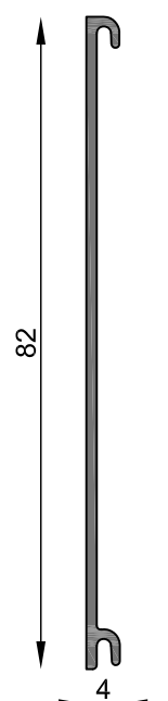
MT-0898 Tapa zócalo Peso estimado: 0.319 Kg/m Largo STD: 6030 mm
