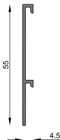
MT-2790 Tapa zócalo pasa cables Peso estimado: 0.232 Kg/m Largo STD: 6030 mm
