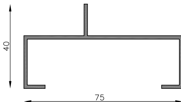
MT-2448 Canal aletado Peso estimado: 0.664 Kg/m Largo STD: 6030 mm
