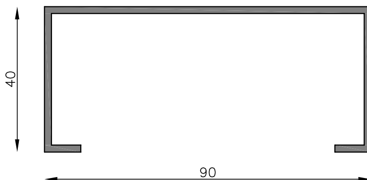
MT-2449 Canal liso 90 x 40 mm Peso estimado: 0.937 Kg/m Largo STD: 6030 mm
