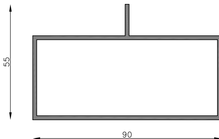
MT-2451 Tubo aletado 90 x 40 mm Peso estimado: 1.372 Kg/m Largo STD: 6030 mm
