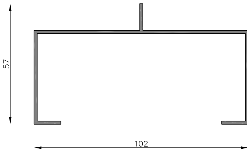
TO-0840 Canal de una ceja Peso estimado: 0.902 Kg/m Largo STD: 6200 mm
