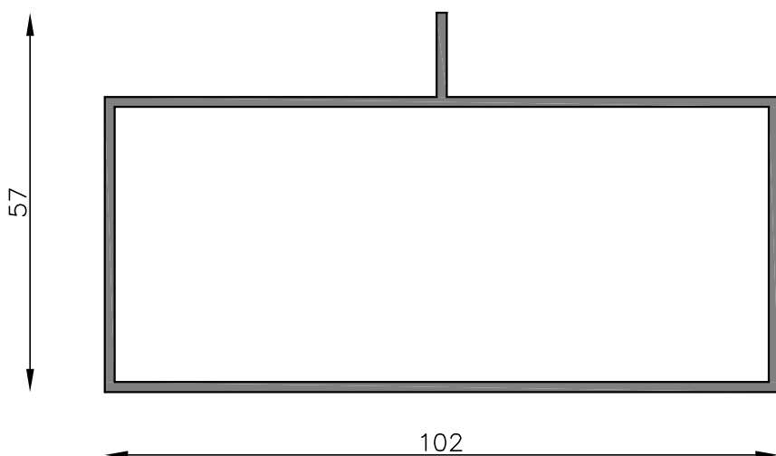
TO-1033 Una ceja centrada Peso estimado: 1.210 Kg/m Largo STD: 6200 mm
