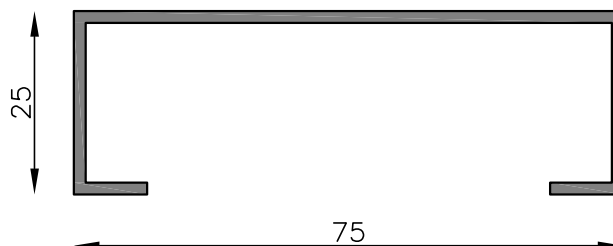
MT-2454 Canal liso - 75 x 25 mm Peso estimado: 0.599 Kg/m Largo STD: 6030 mm
