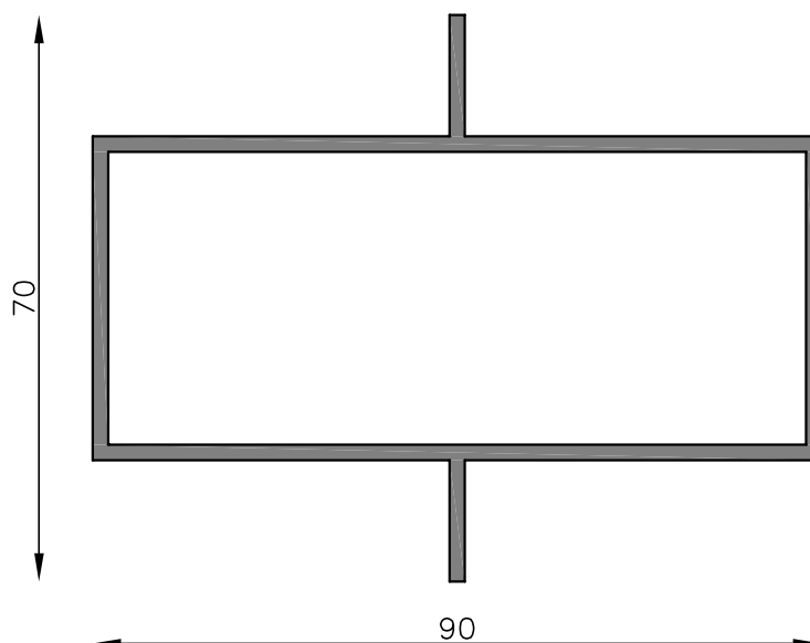
MT-2452 Tubo aletado - 90 x 40 mm Peso estimado: 1.450 Kg/m Largo STD: 6030 mm
