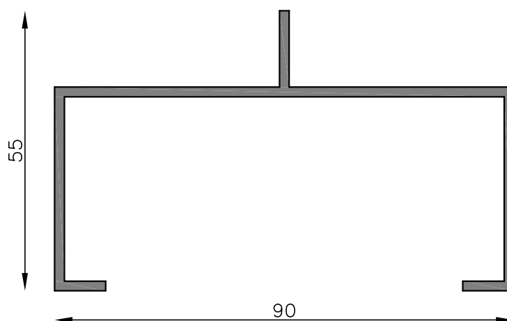
MT-2450 Canal aletado 90 x 40 mm Peso estimado: 1.013 Kg/m Largo STD: 6030 mm
