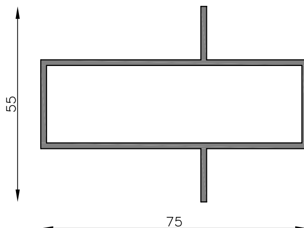
MT-2455 Tubo aletado - 75 x 25 mm Peso estimado: 0.967 Kg/m Largo STD: 6030 mm
