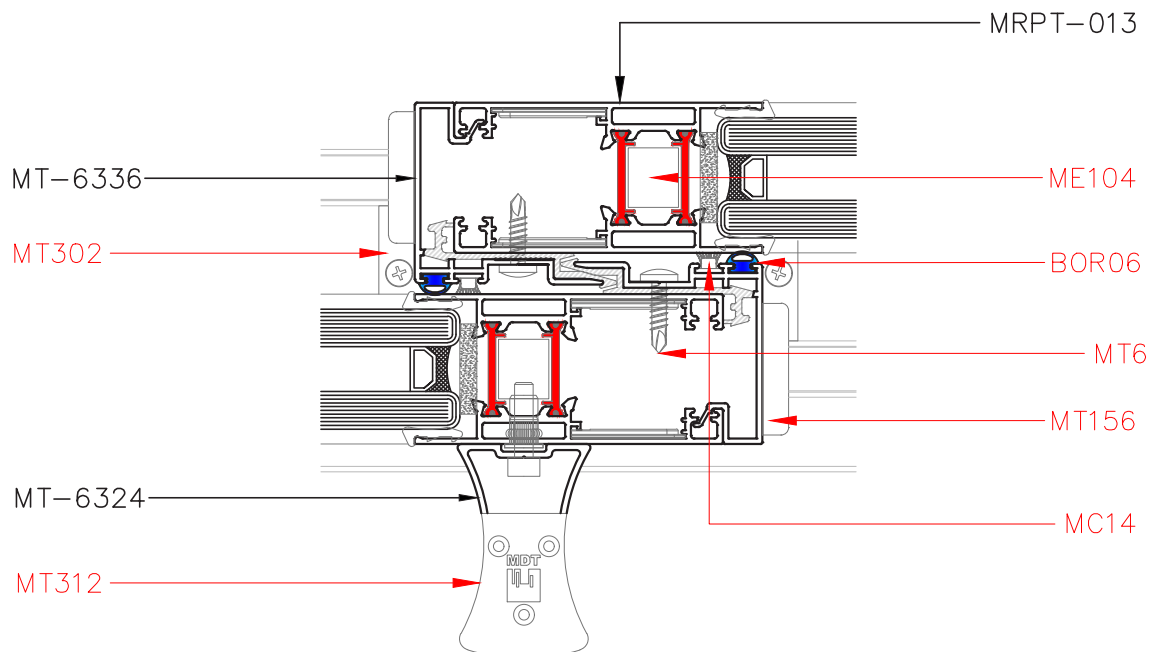
Corte 4-4
