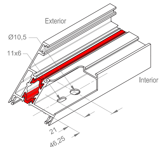
Mecanizado de marco para escuadra ME101
