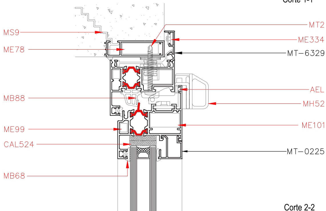
Corte 1-1
