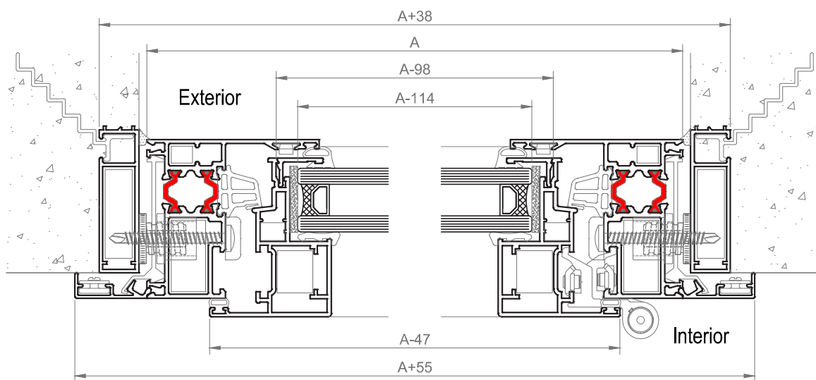
Corte 3 - 3
