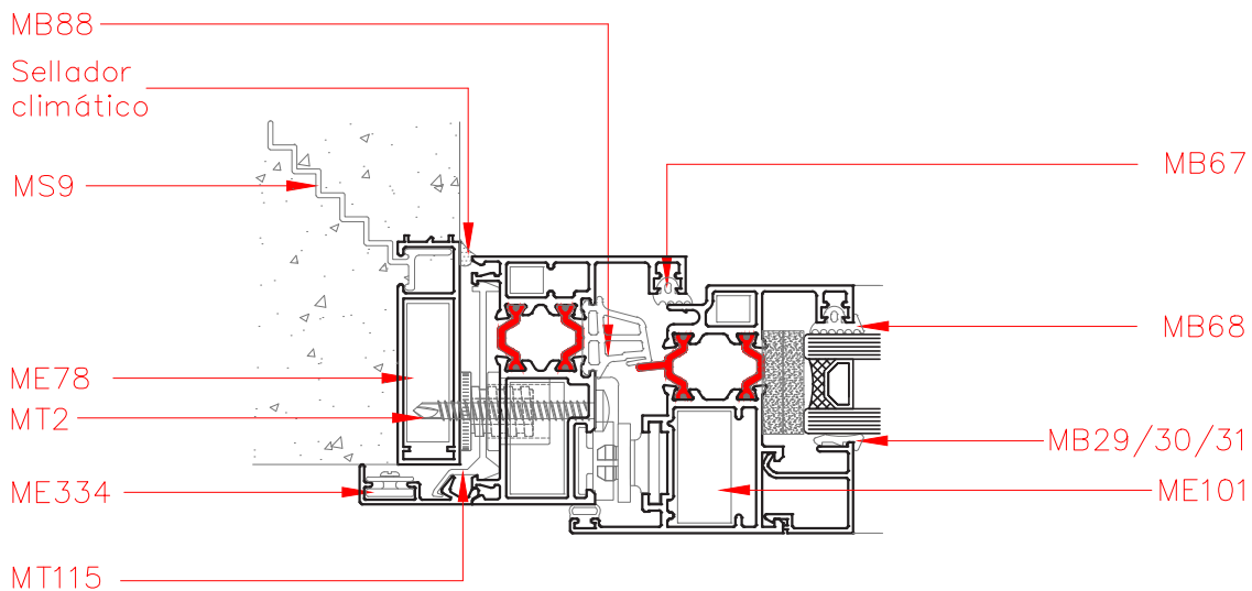
Corte 3-3
