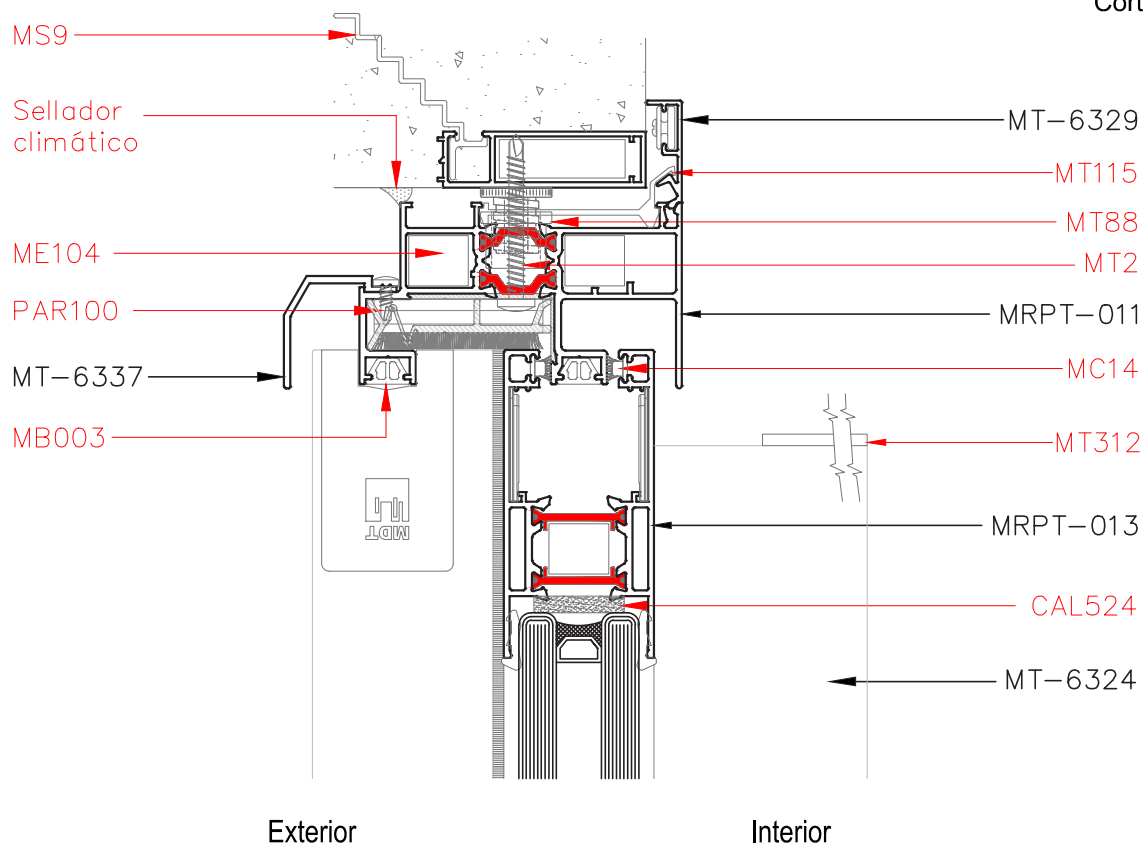
Corte 1-1
