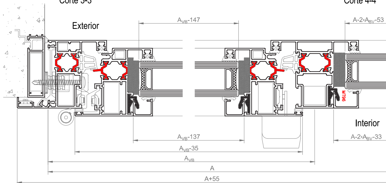
Corte 3-3
