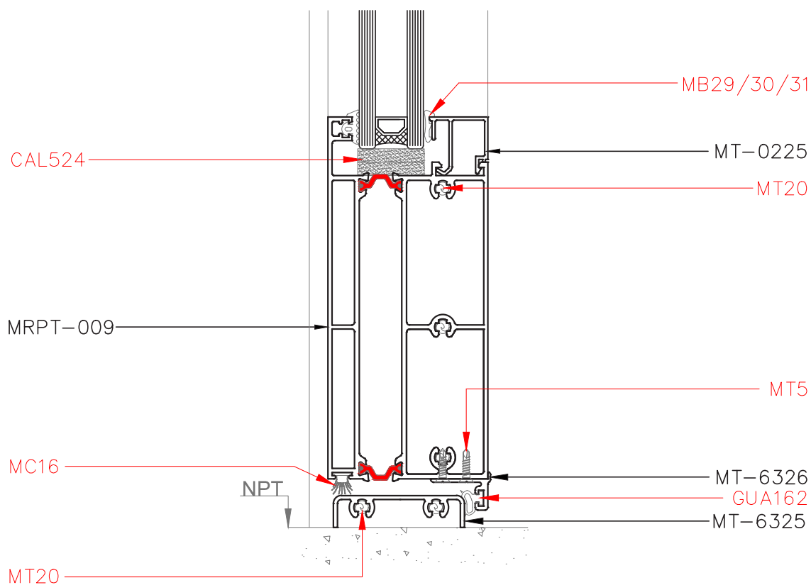
Corte 2-2
