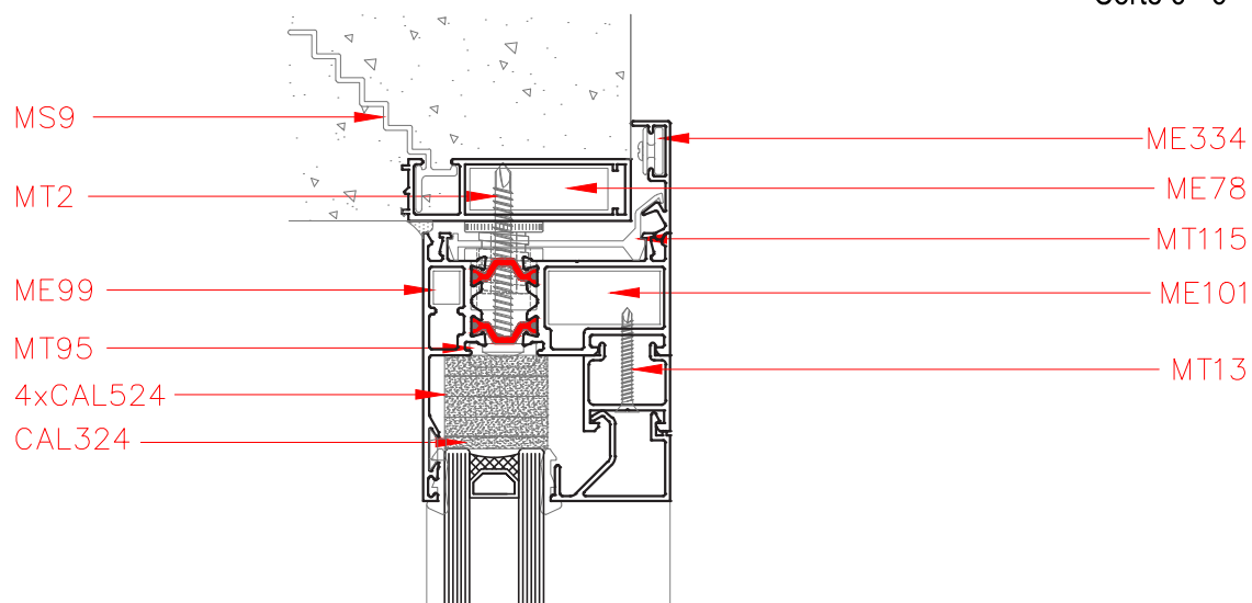
Corte 6 - 6
