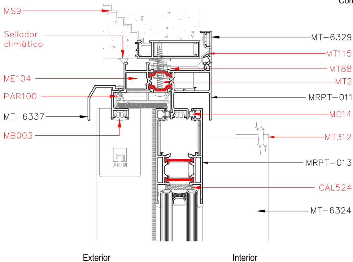
Corte 1-1
