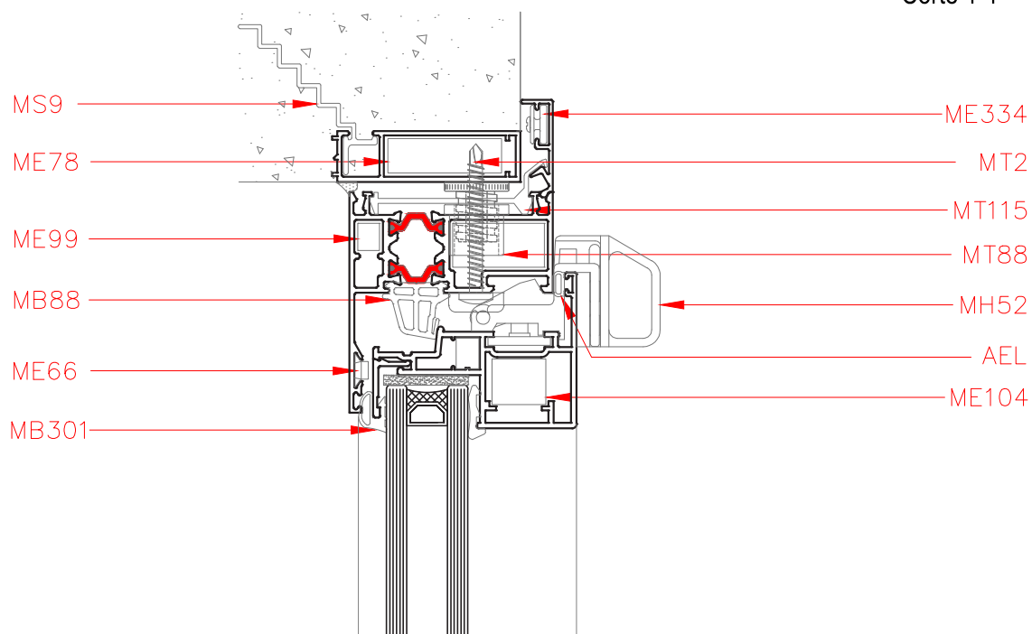
Corte 2 - 2
