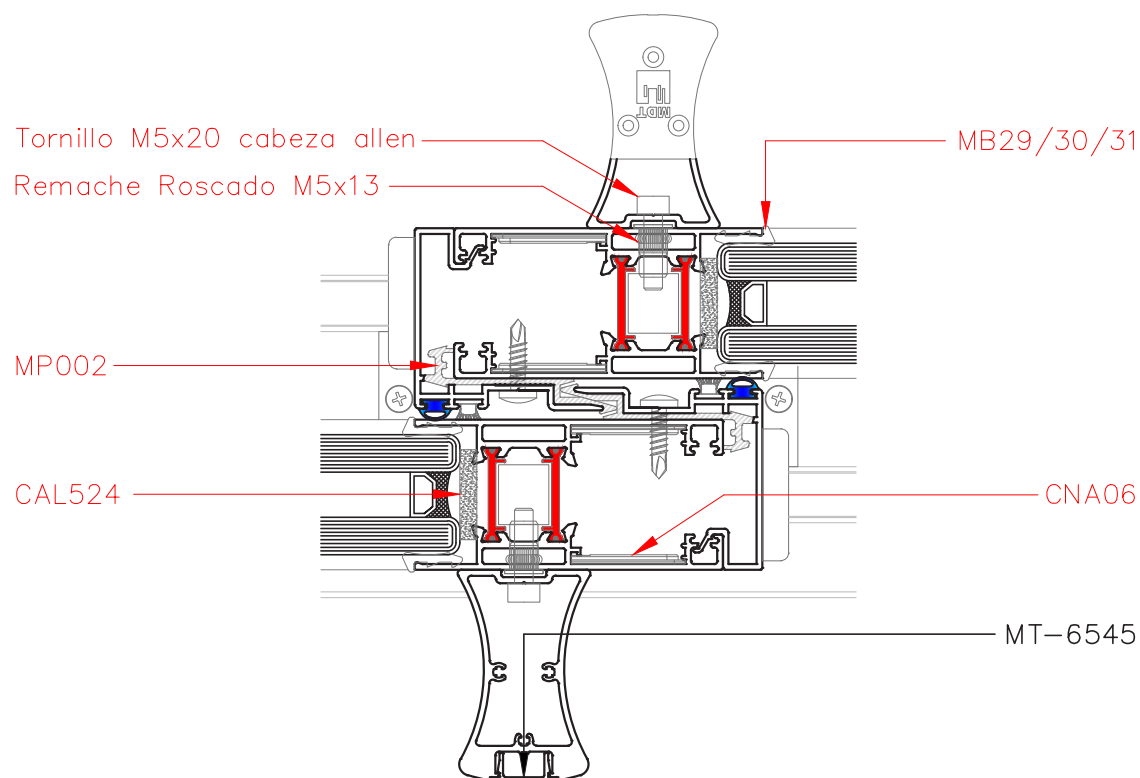
Corte 4-4 / 5-5
