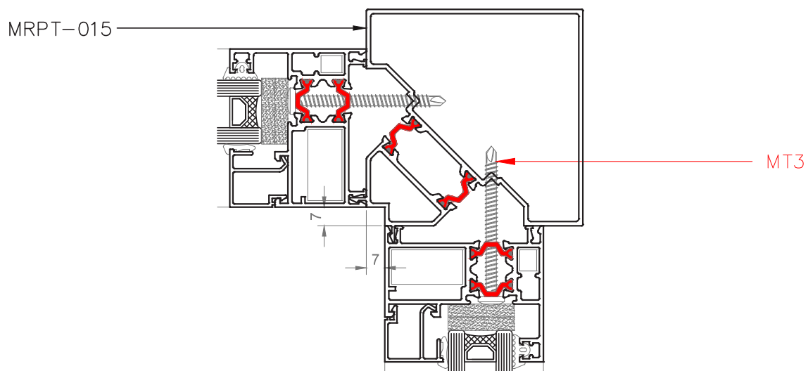
Acople a 90° con módulo 75mm
