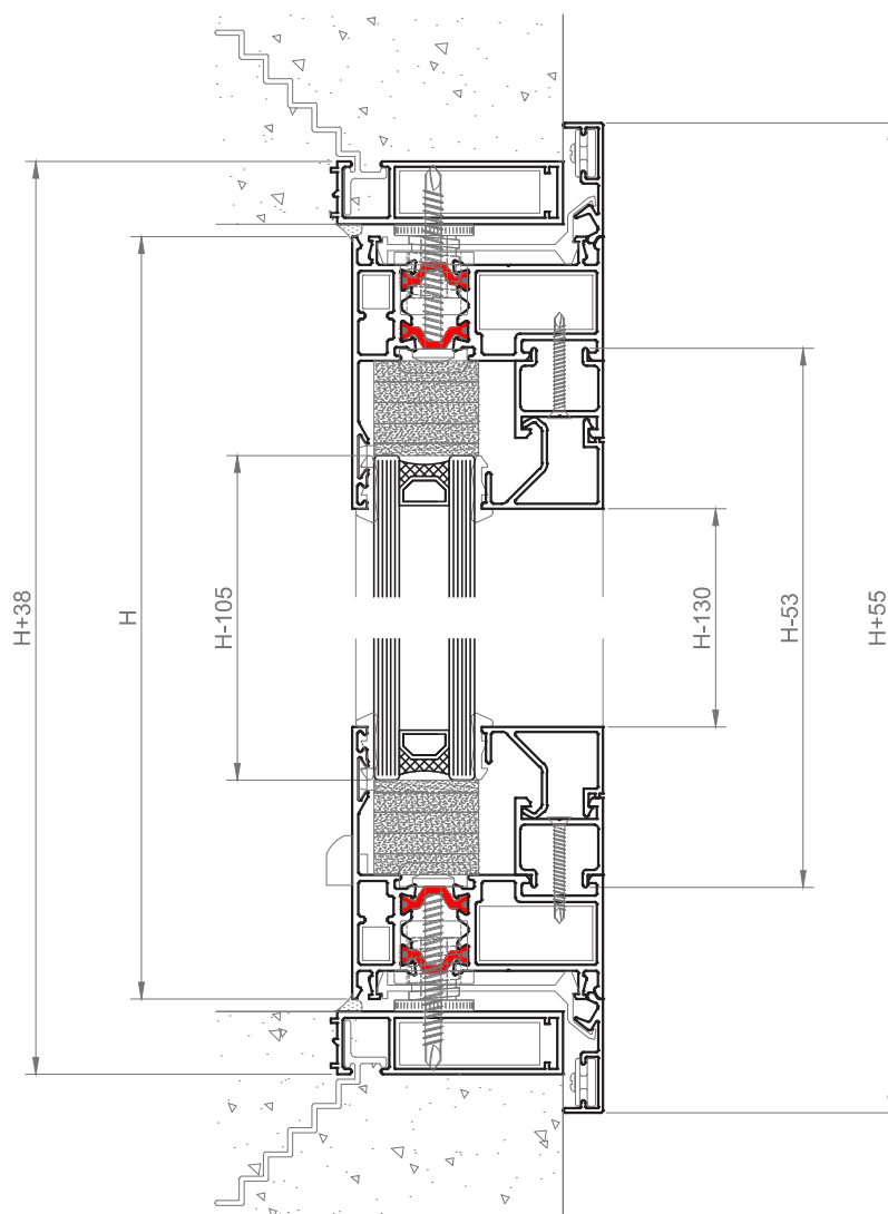
Corte 7 - 7
