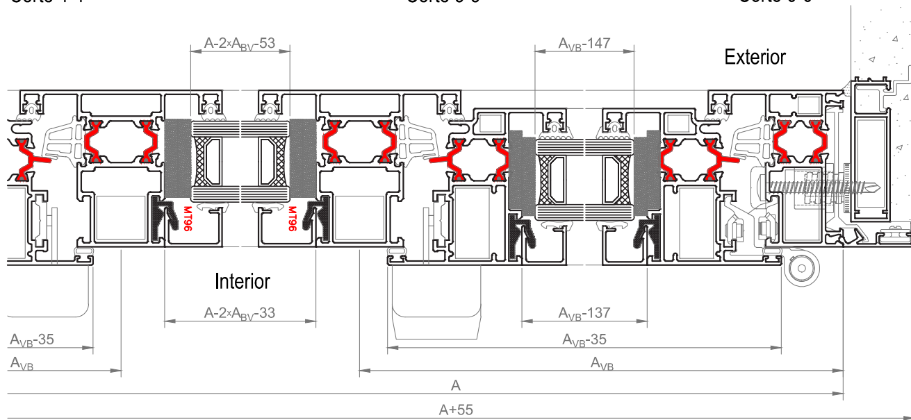
Corte 4-4
