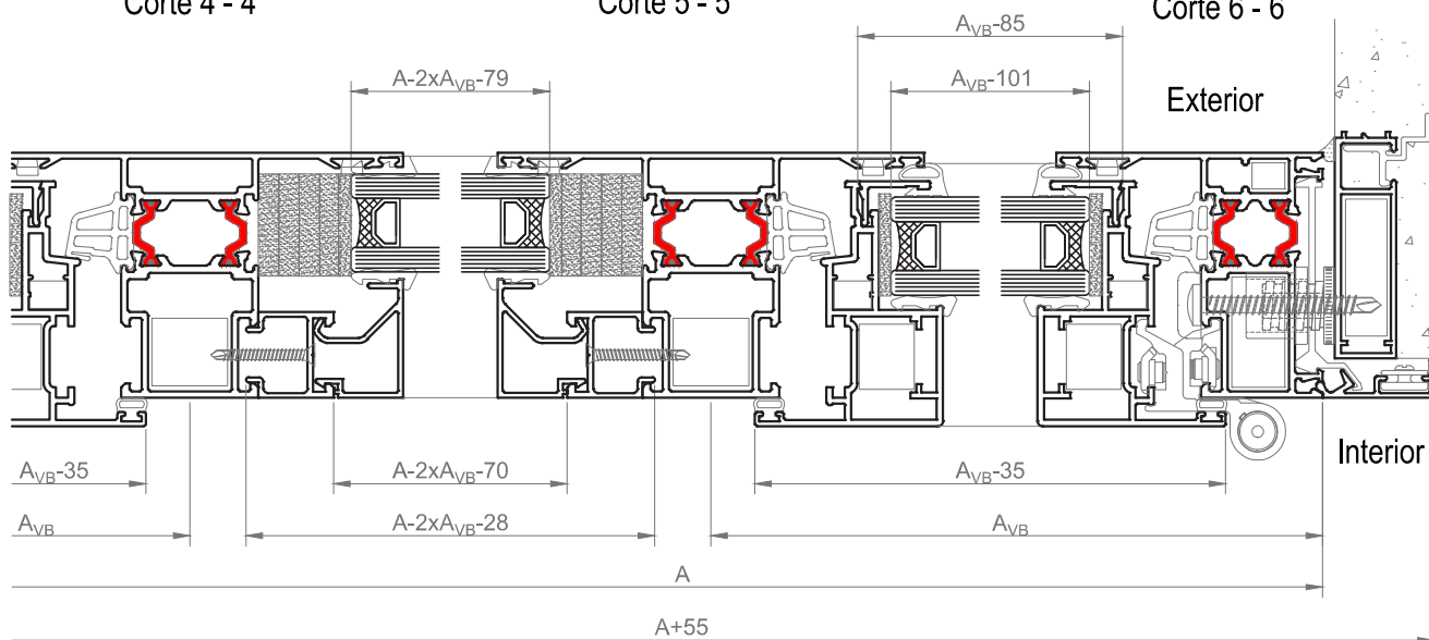
Corte 4 - 4
