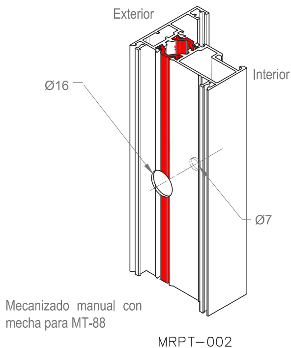
Mecanizado para MT88
