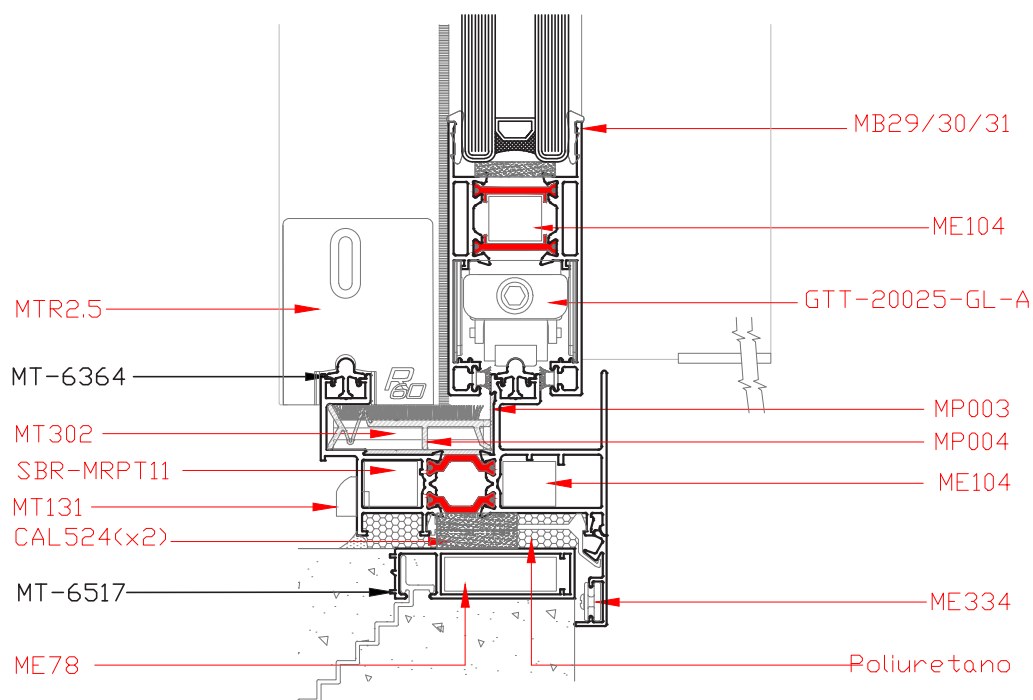
Corte 2-2
