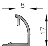
MT-0233 Contravidrio curvo interior 8mm Peso estimado: 0.135 Kg/m Largo STD: 6030 mm
