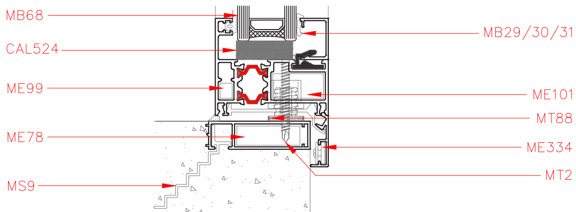
Corte 7 - 7
