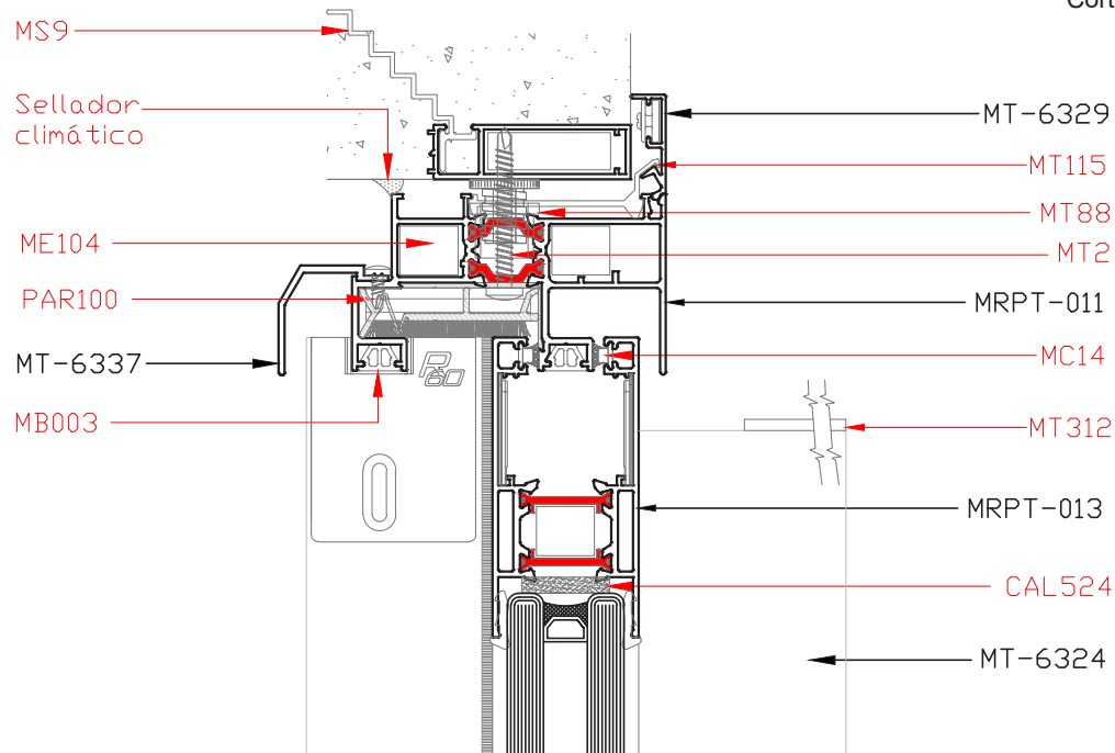
Corte 1-1
