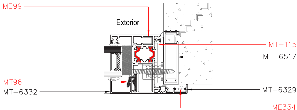
Corte 6 - 6
