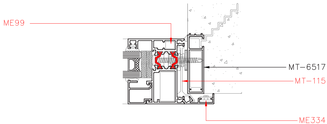
Corte 6 - 6
