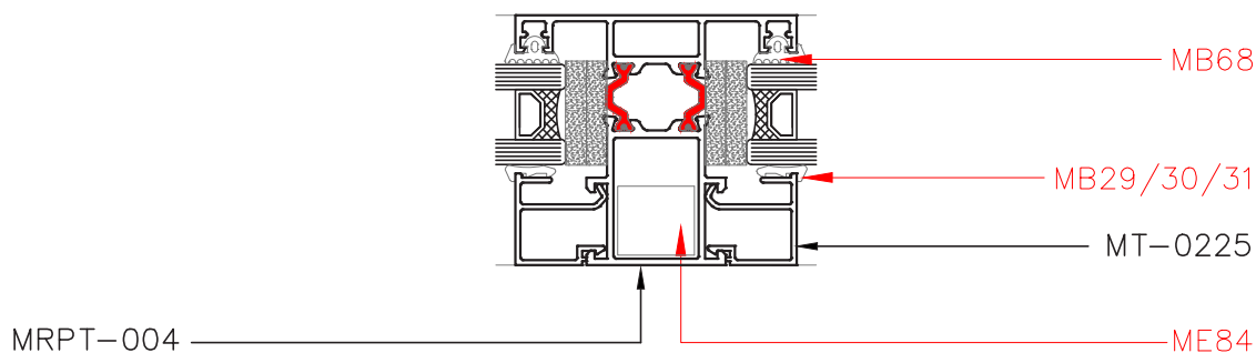
Corte 6 - 6
