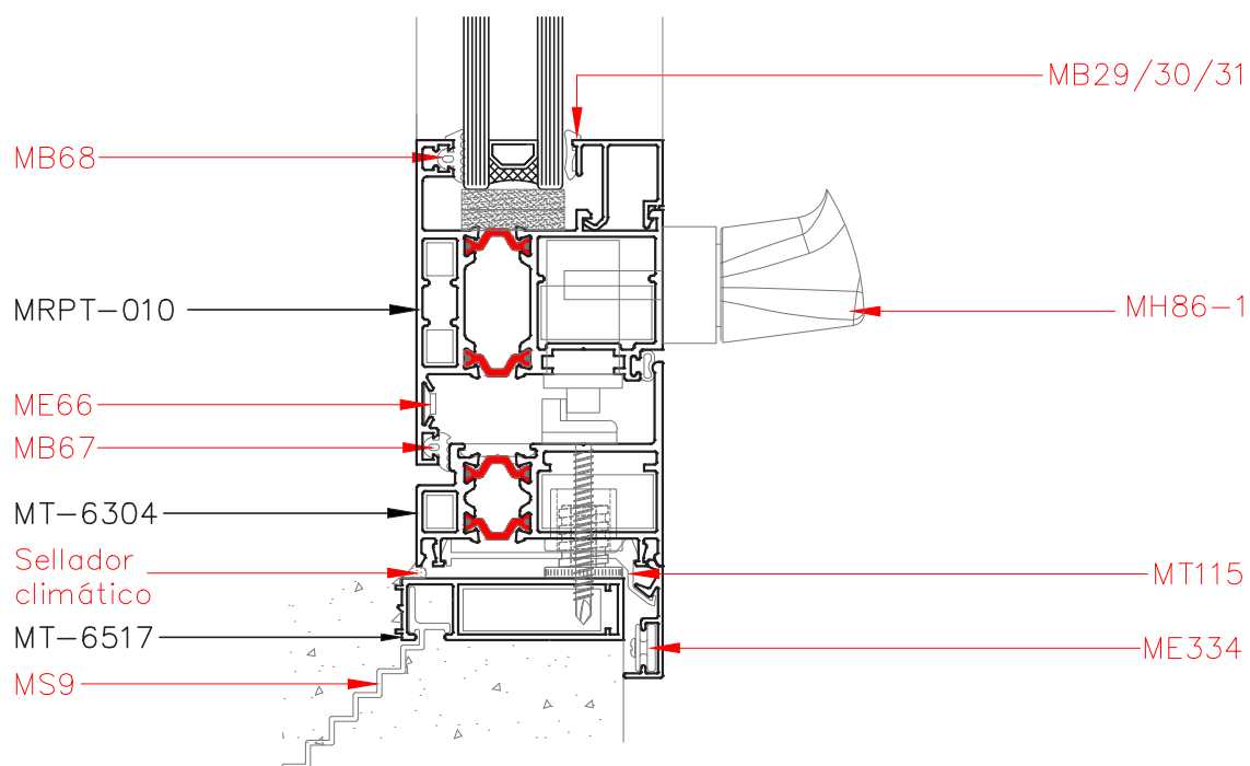
Corte 2-2
