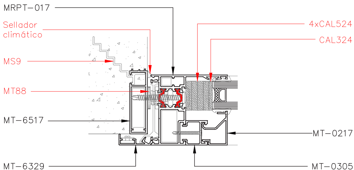
Corte 4-4
