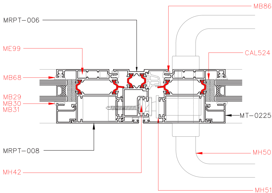
Corte 6-6
