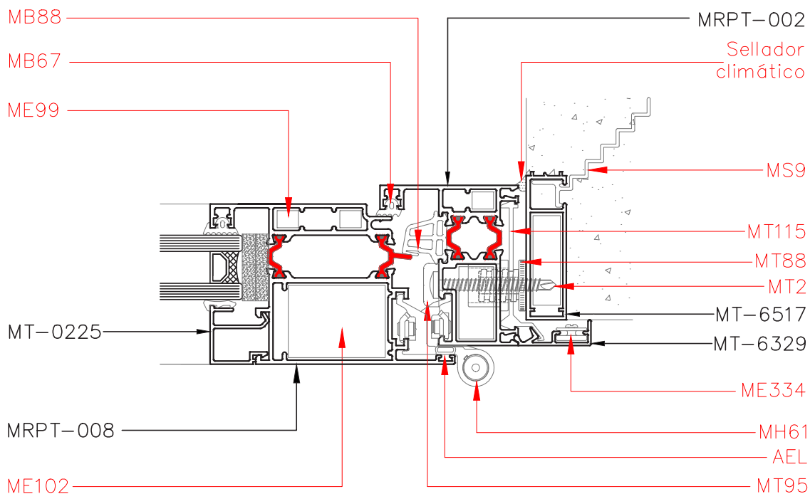
Corte 4-4
