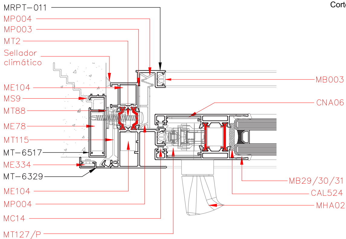
Corte 4-4
