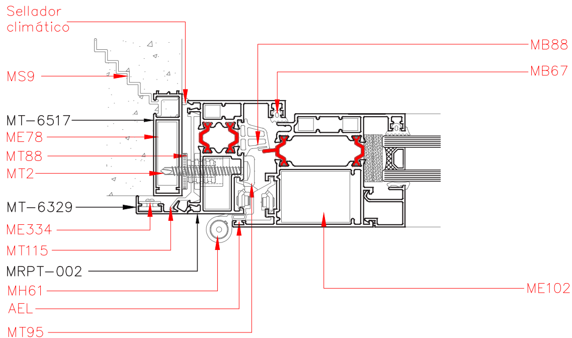
Corte 5-5
