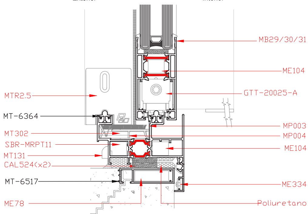
Corte 2-2
