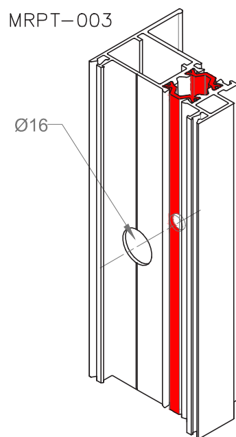
Mecanizado para MT88
