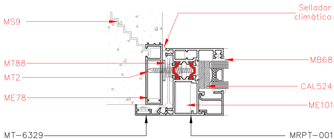
Corte 4-4
