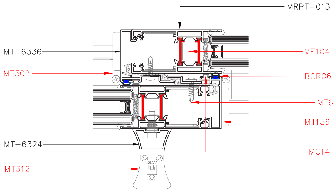
Corte 4-4 / 5-5
