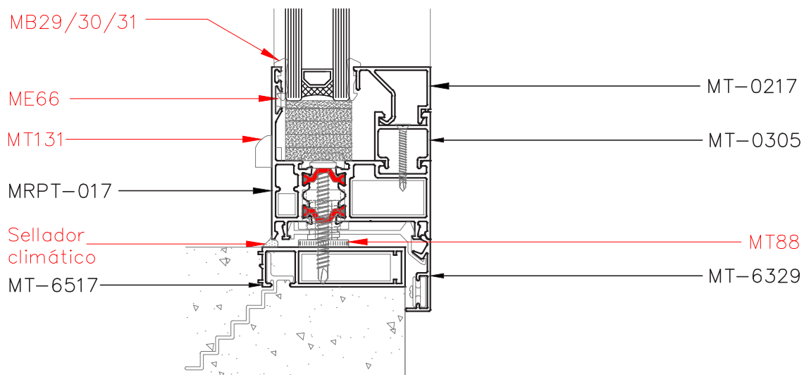
Corte 3 - 3
