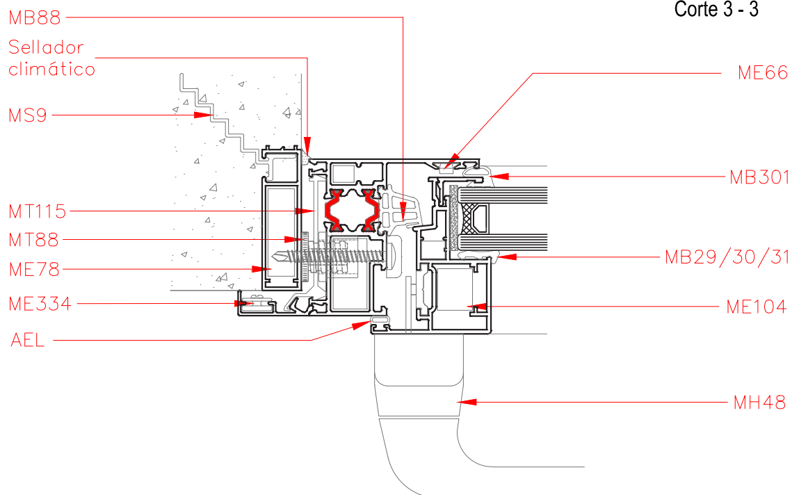
Corte 3 - 3
