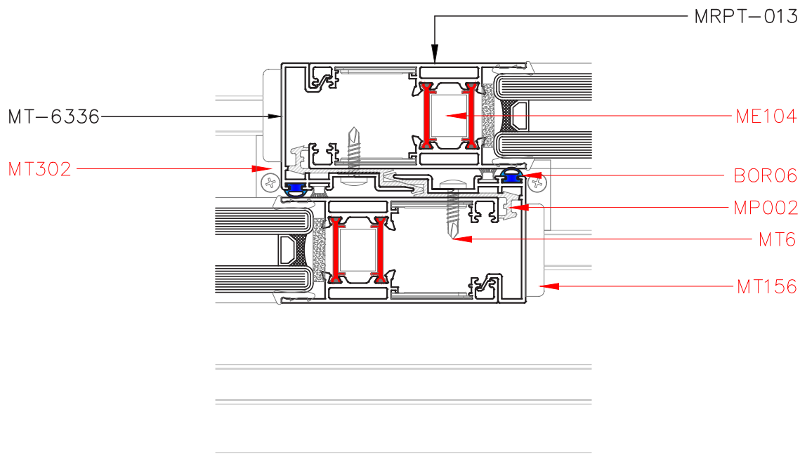
Corte 6-6
