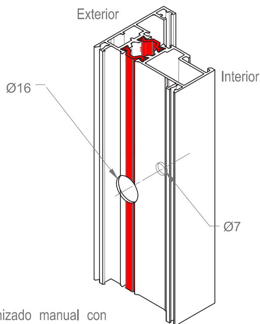
Mecanizado para MT88
