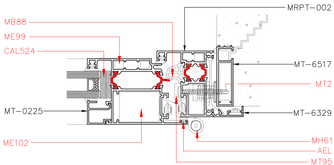
Corte 4-4
