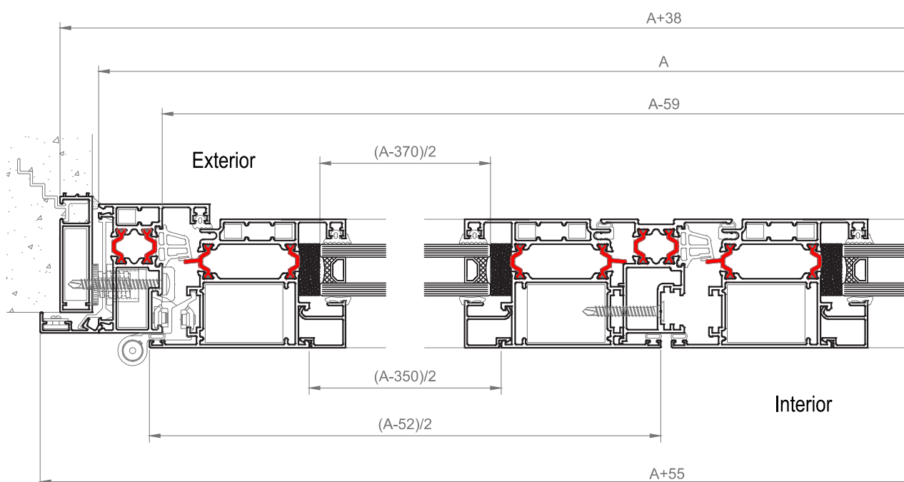
Corte 5-5
