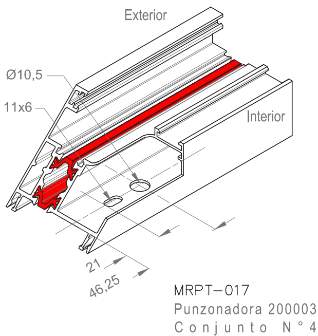
Mecanizado de marco para escuadra ME101
