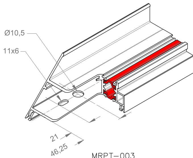
Mecanizado de pletina para accesorios
