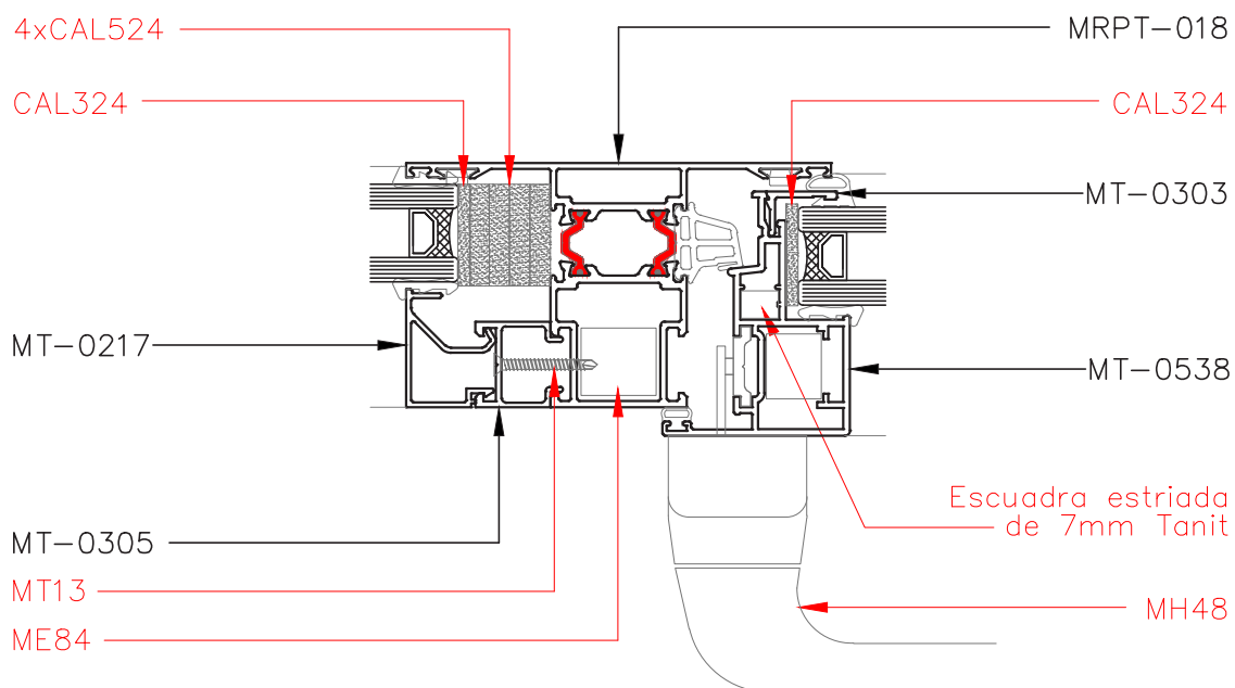
Corte 5 - 5
