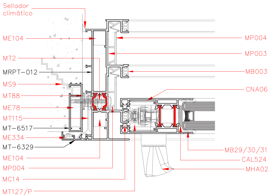
Corte 3-3
