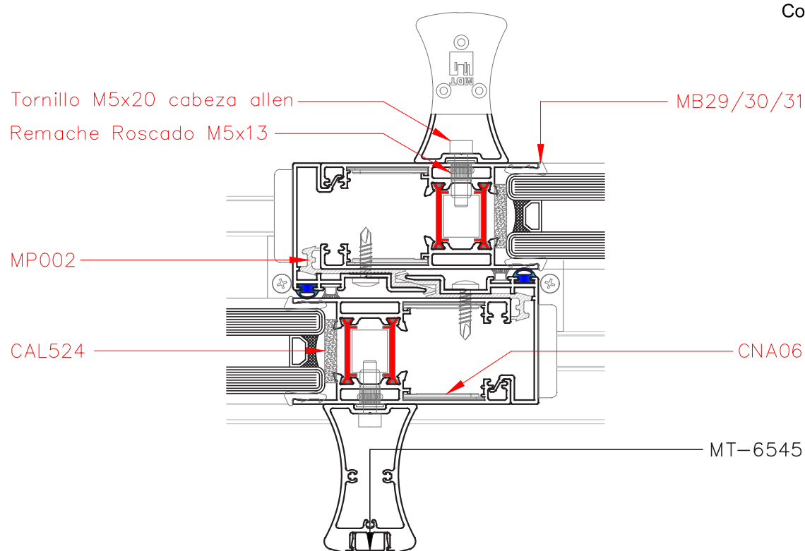
Corte 4-4
