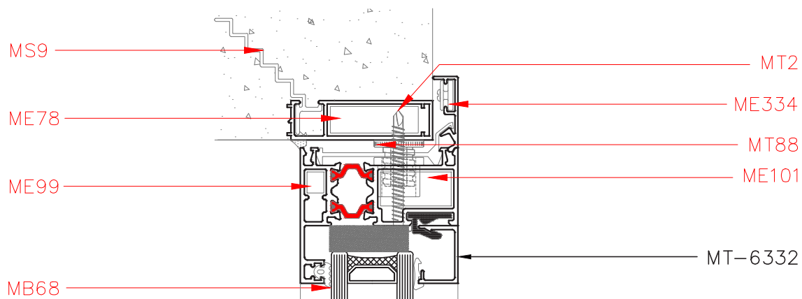
Corte 6 - 6
