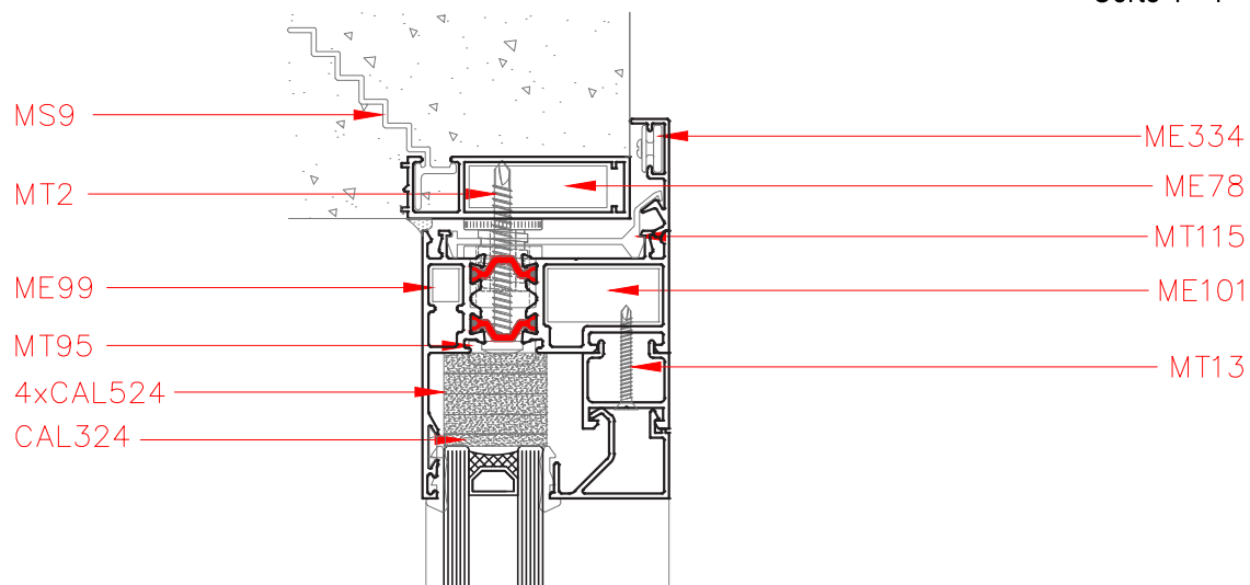
Corte 1 - 1
