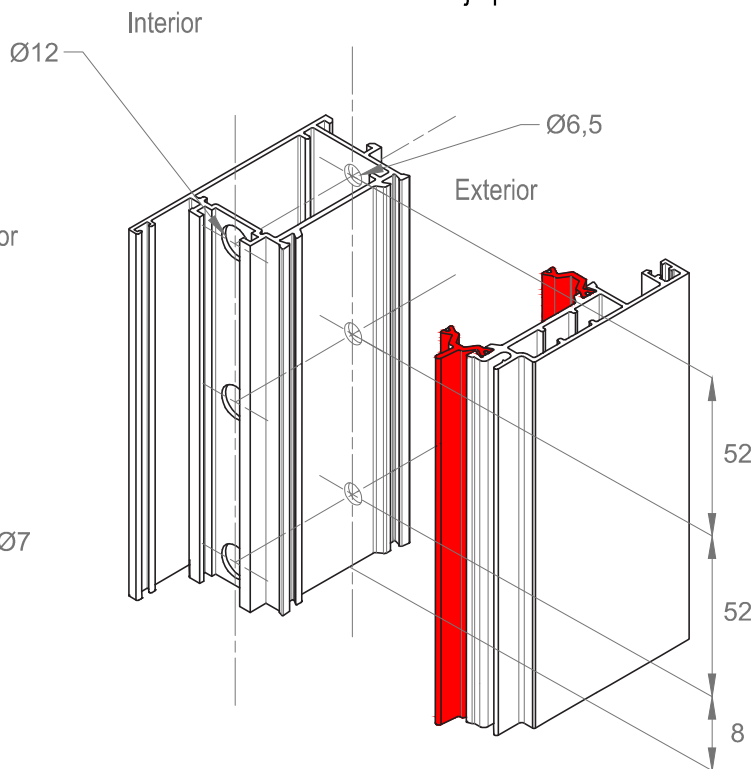
Mecanizado de hoja para zócalo
