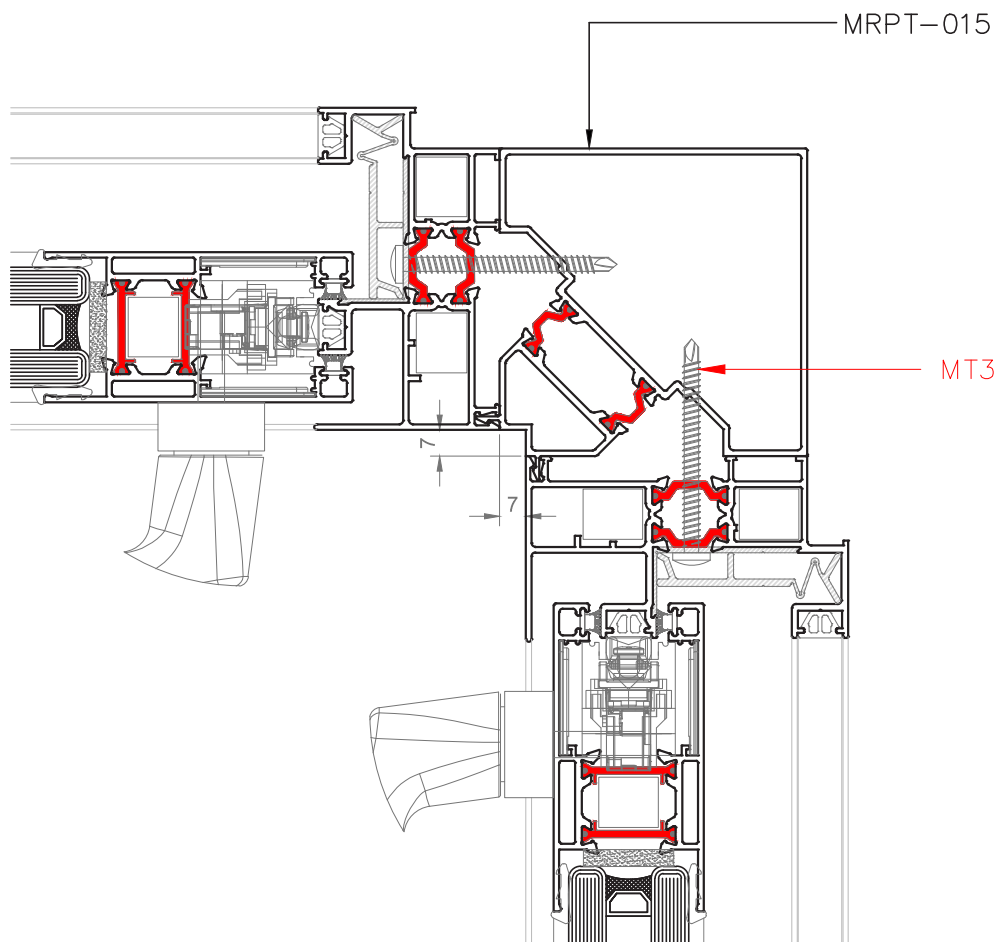
Acople a 90° con módulo 75mm
