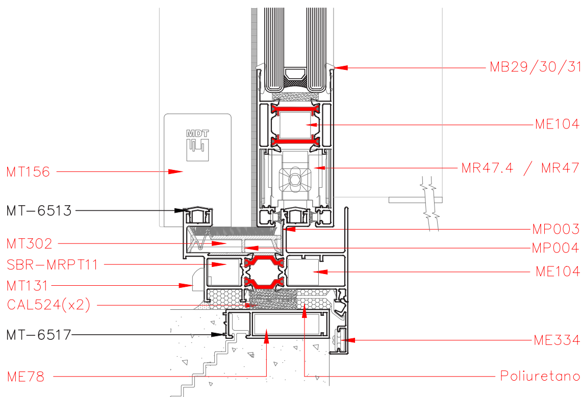
Corte 2-2
