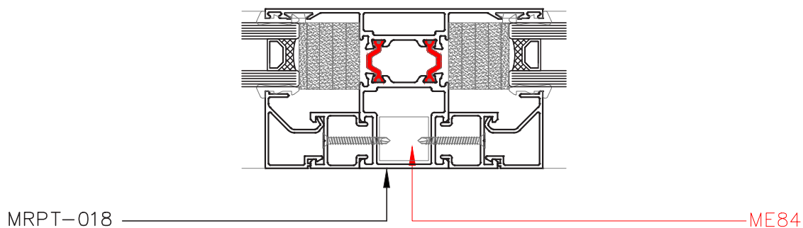
Corte 5 - 5
