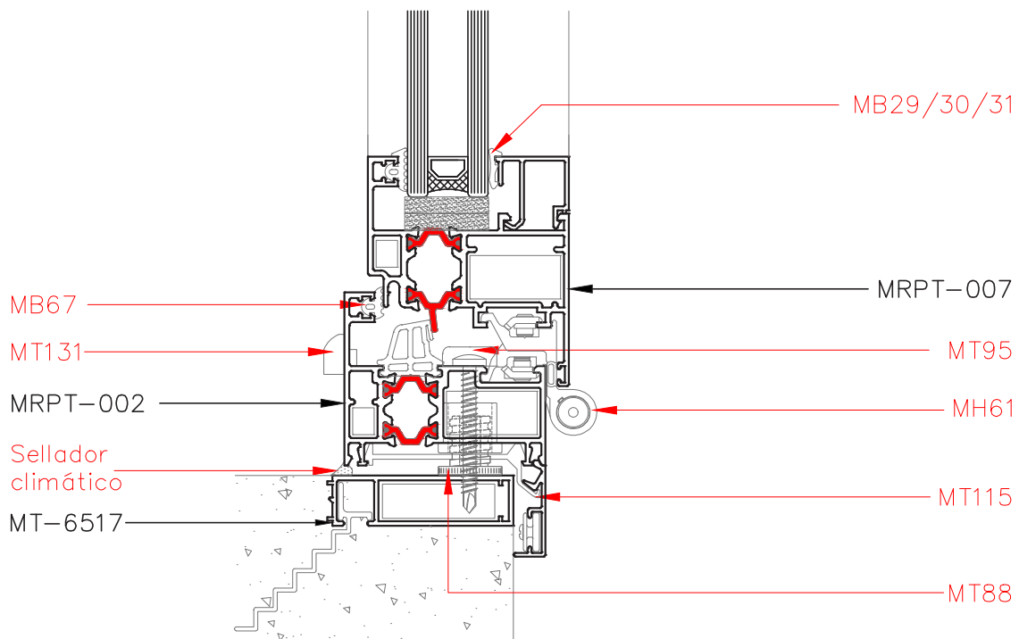
Corte 2-2
