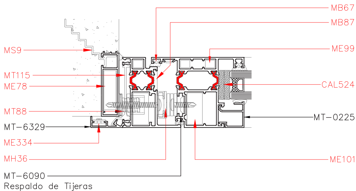
Corte 3-3
