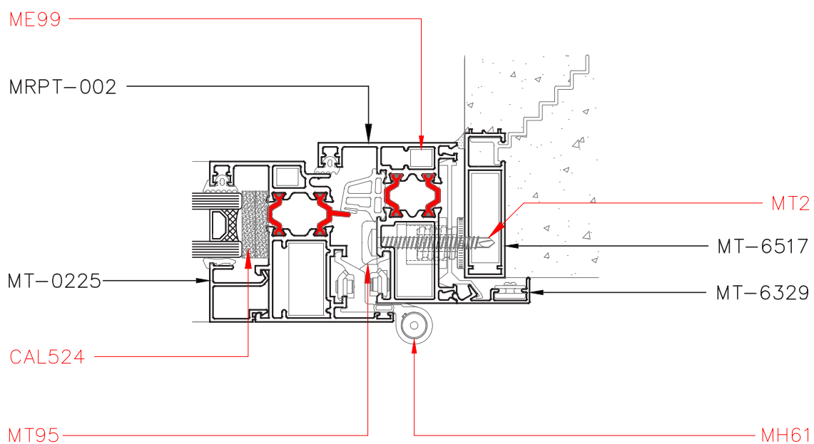
Corte 4 - 4
