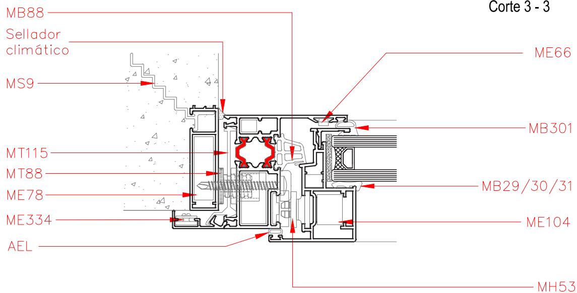
Corte 3 - 3
