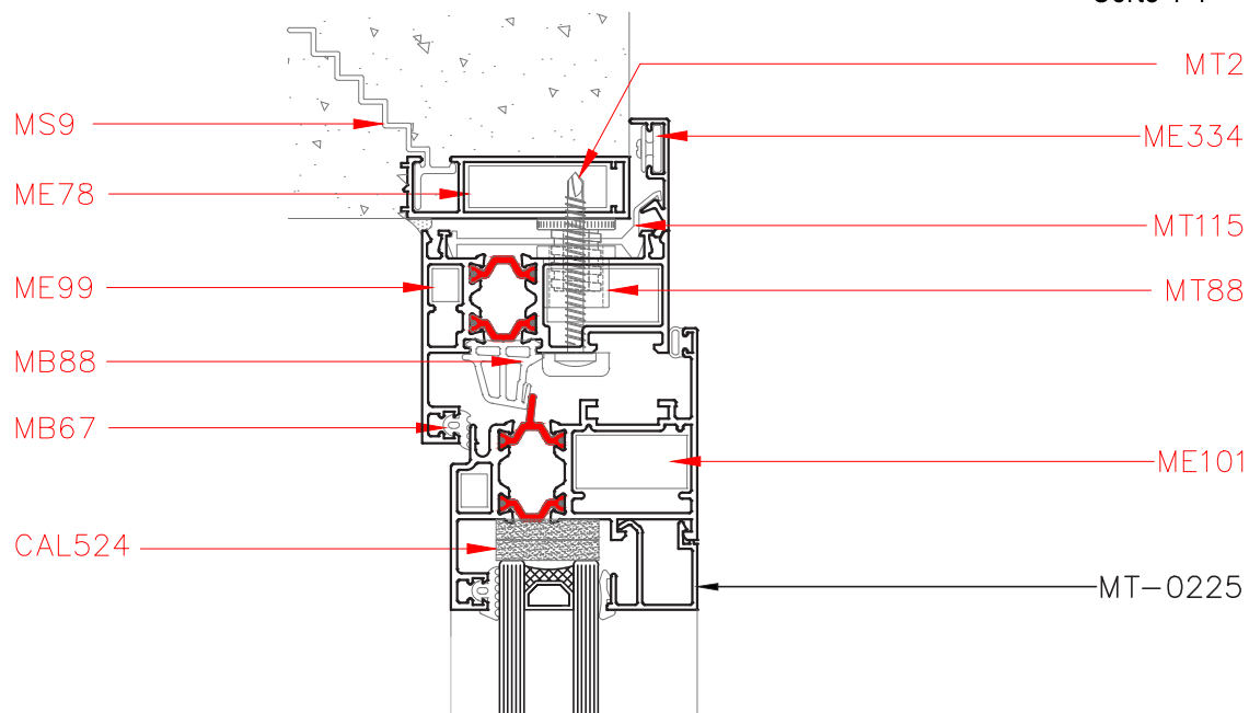
Corte 1-1
