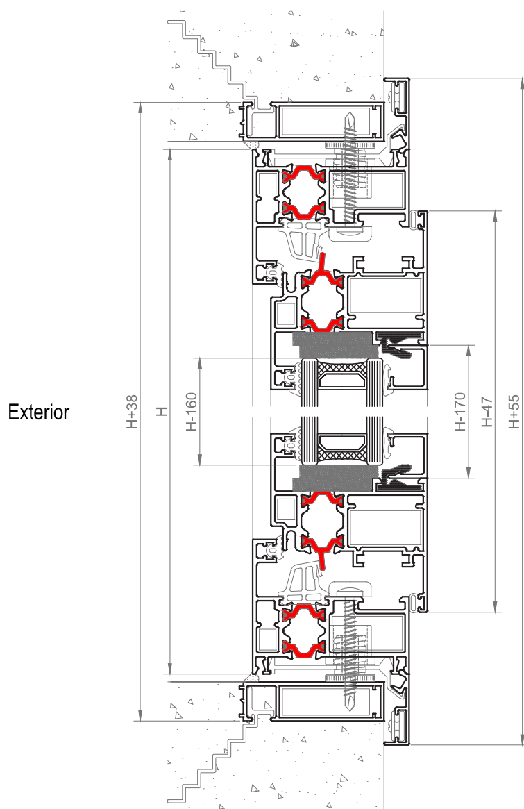
Corte 3-3
